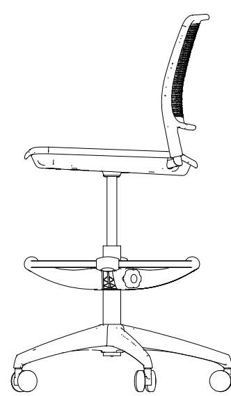
Task Stool
